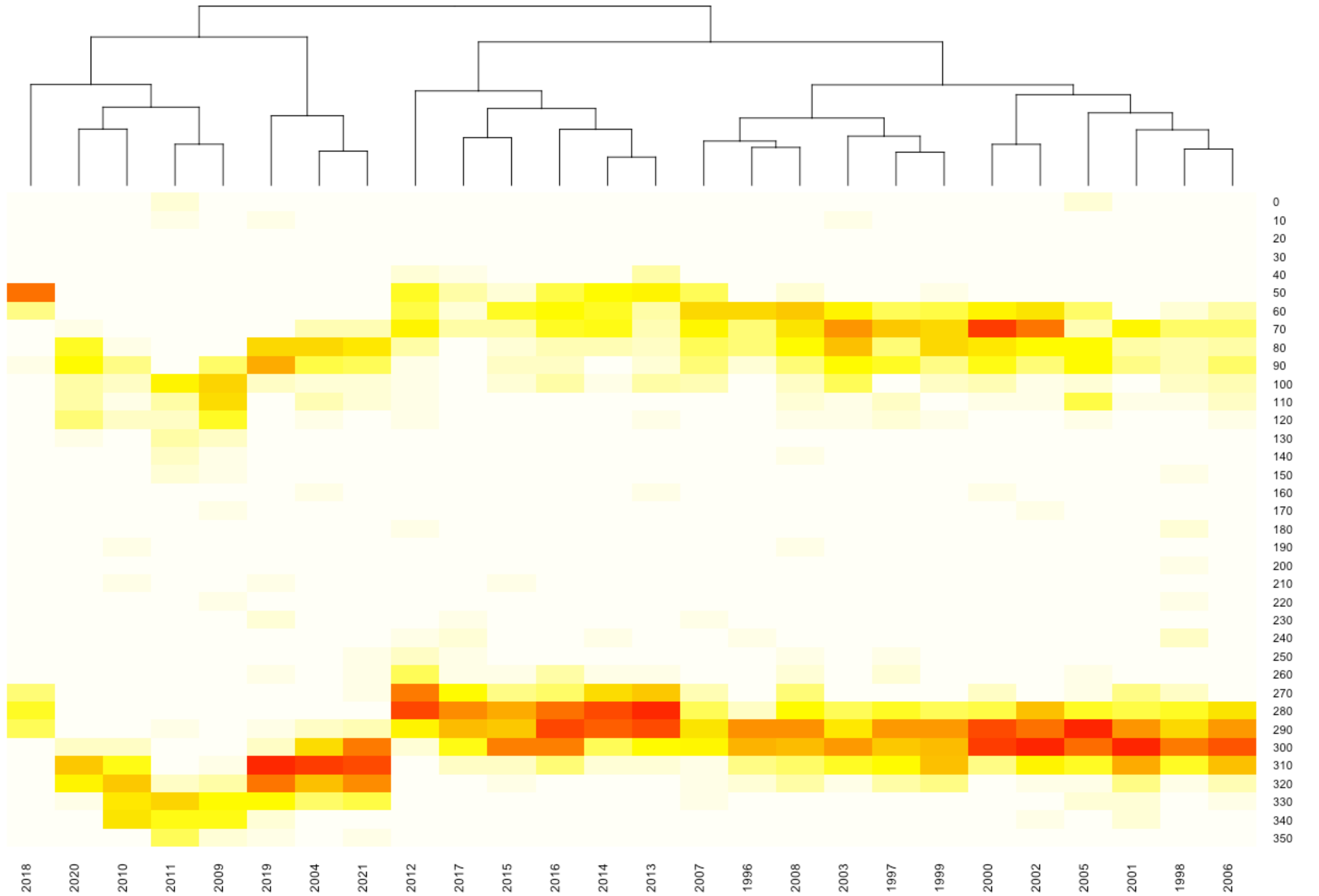
Vents période pascale force 5 ou plus (nombre de tranches de 3h) en fonction de la direction Station de Cap Cepet
