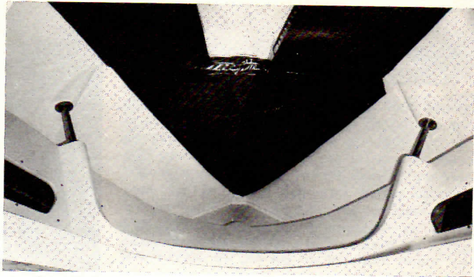
L'effort du mât est supporté par un arceau qui évite d'encombrer la petite cabine par une épontille.
