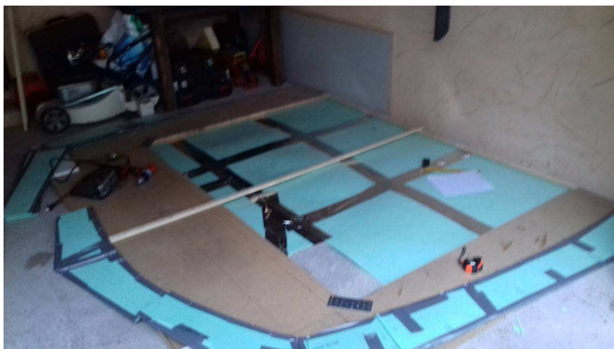
Report des plans de pont sur gabarit en bois
