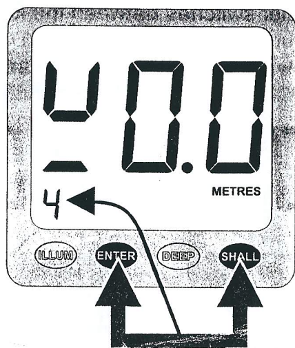
Figure 10 : Réglage de l'indice de fréquence.
