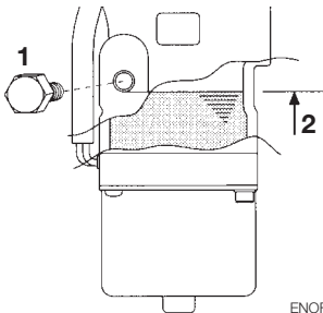
1. Bouchon d'huile 2. Niveau d'huile
