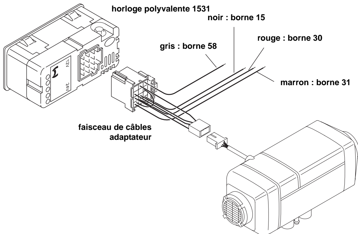
Fig. 708 Raccordement schématique de l'horloge polyvalente
