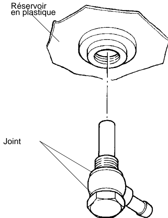
Fig. 803 Prélèvement de carburant dans un réservoir en plastique (prélèvement via le bouchon de décharge du réservoir)
