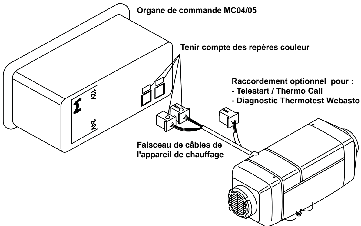
Fig. 709 Raccordement schématique de l'élément de commande MC04/05
