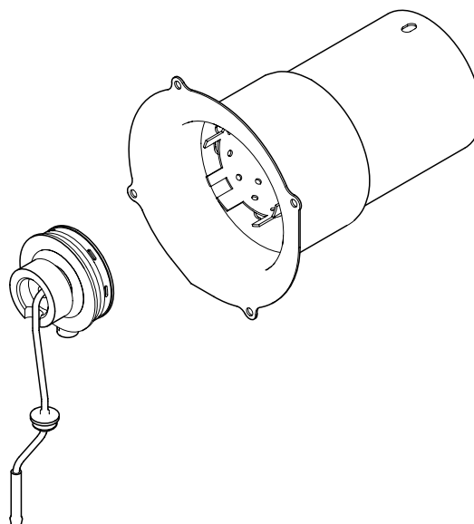
Insert de brûleur (diesel) et tuyau de combustion
