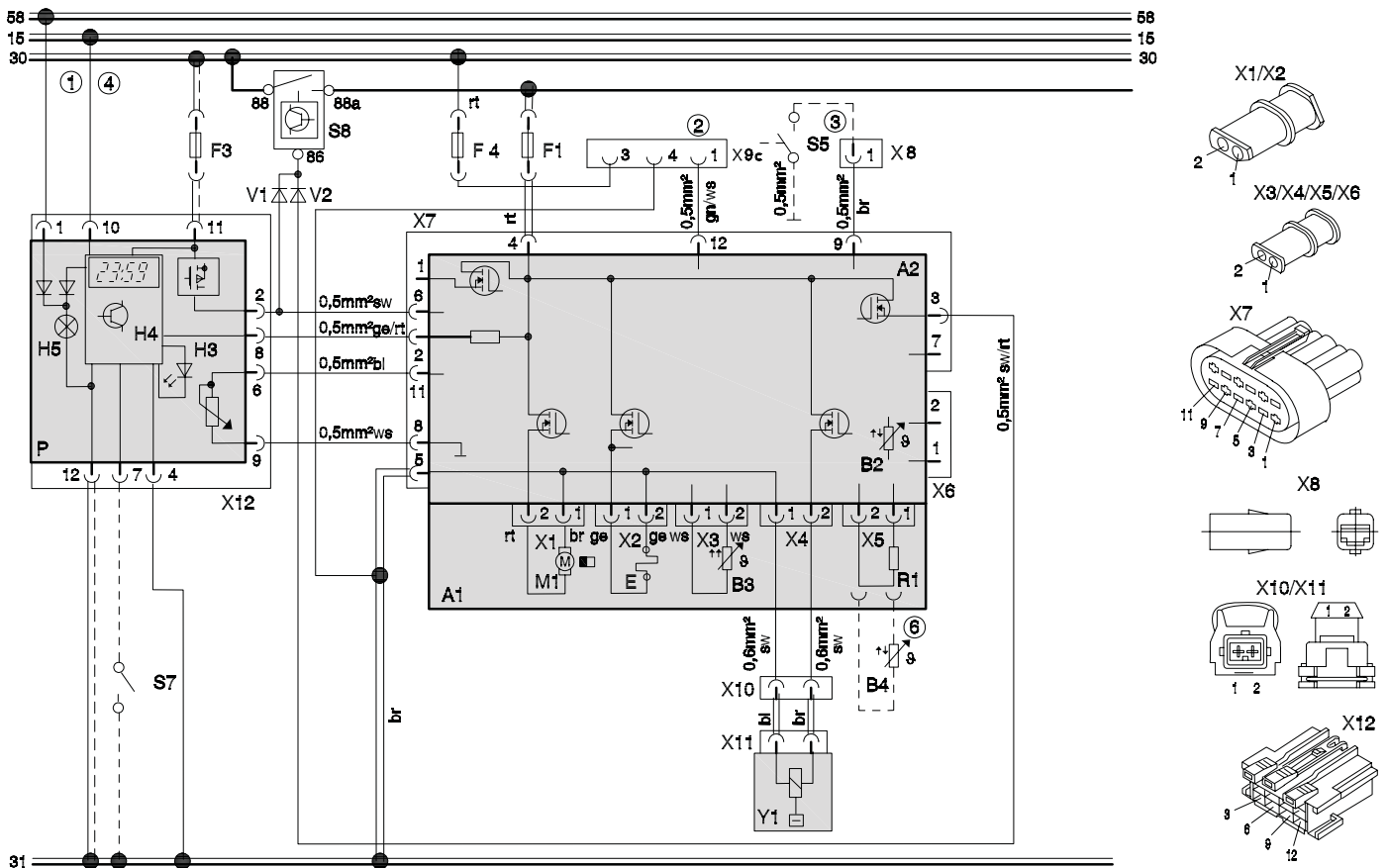
Fig. 705 Schéma électrique d'ensemble (diesel) 12V/24V, avec horloge polyvalente et coupe-batterie électrique
