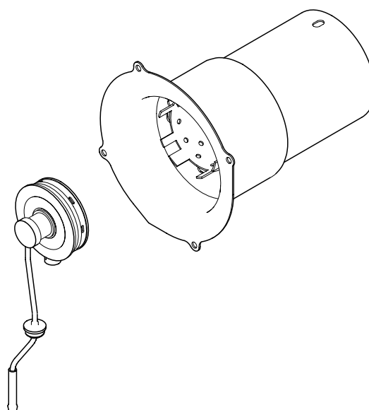
Insert de brûleur (essence) et tuyau de combustion
