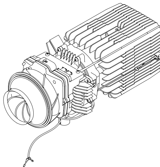
Appareil de chauffage à air Air Top Evo 3900/5500 sans boîtier
