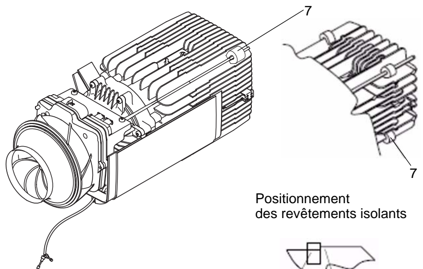
Fig. 901 Extraction / Installation des pièces du boîtier
