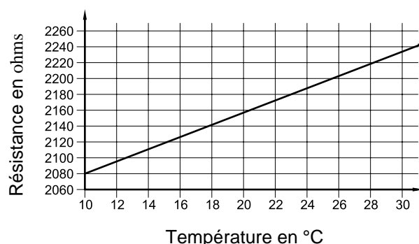
Caractéristiques de résistance d'un capteur de surchauffe PT 2000 à une température comprise entre 10 °C et 30 °C
