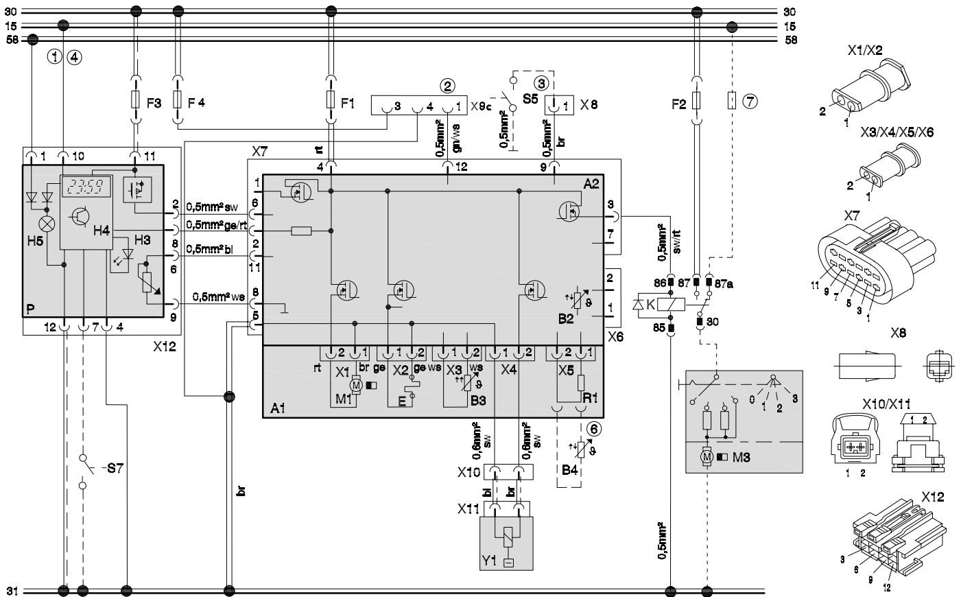
Fig. 704 Schéma électrique d'ensemble 12V/24V, avec horloge polyvalente et soufflante du véhicule
