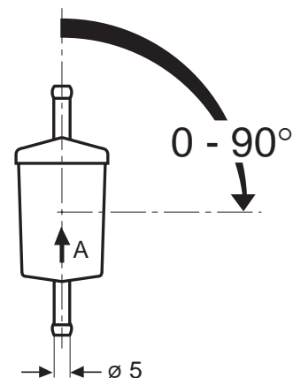
Fig. 807 Filtre à carburant
