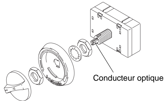
Fig. 812 Élément de commande
