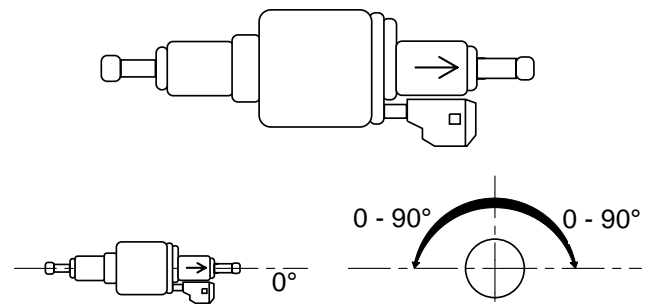
12 volts et 24 volts - diesel DP 30 Position de montage uniquement à l'horizontale
