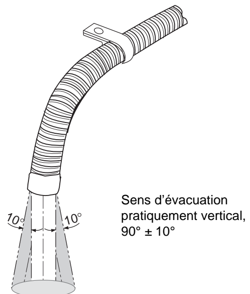
Fig. 809 Embouchure du tuyau d'échappement, position de montage
