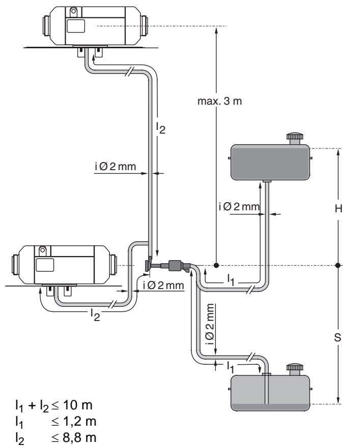
Fig. 801 Alimentation en carburant
