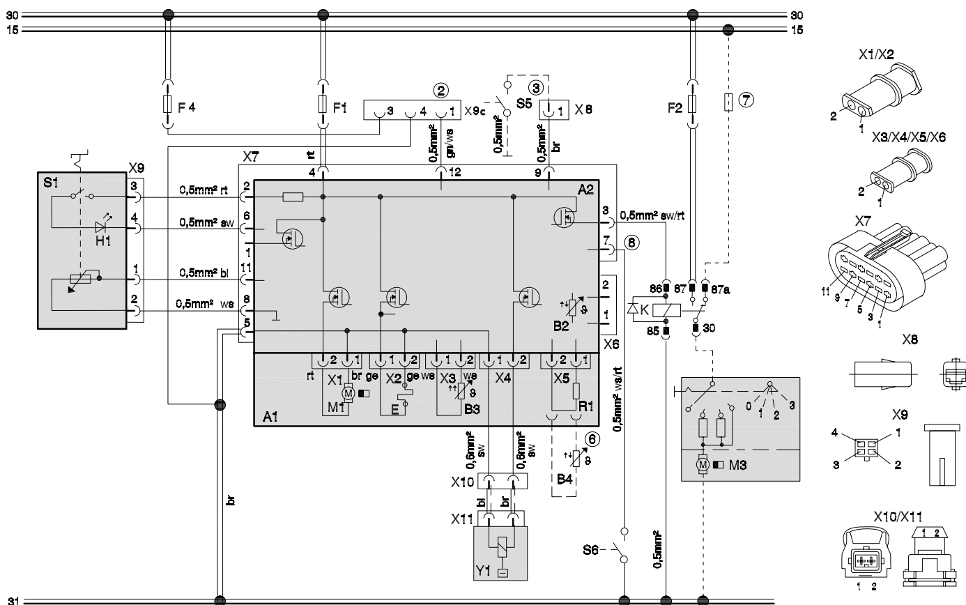
Fig. 702 Schéma électrique d'ensemble 12V/24V, avec élément de commande et soufflante du véhicule
