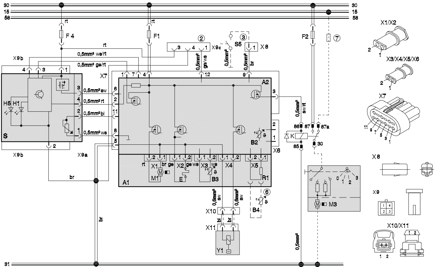
Fig. 706 Schéma électrique d'ensemble (diesel) 12V/24V, avec élément de commande MC04/05 et soufflante du véhicule
