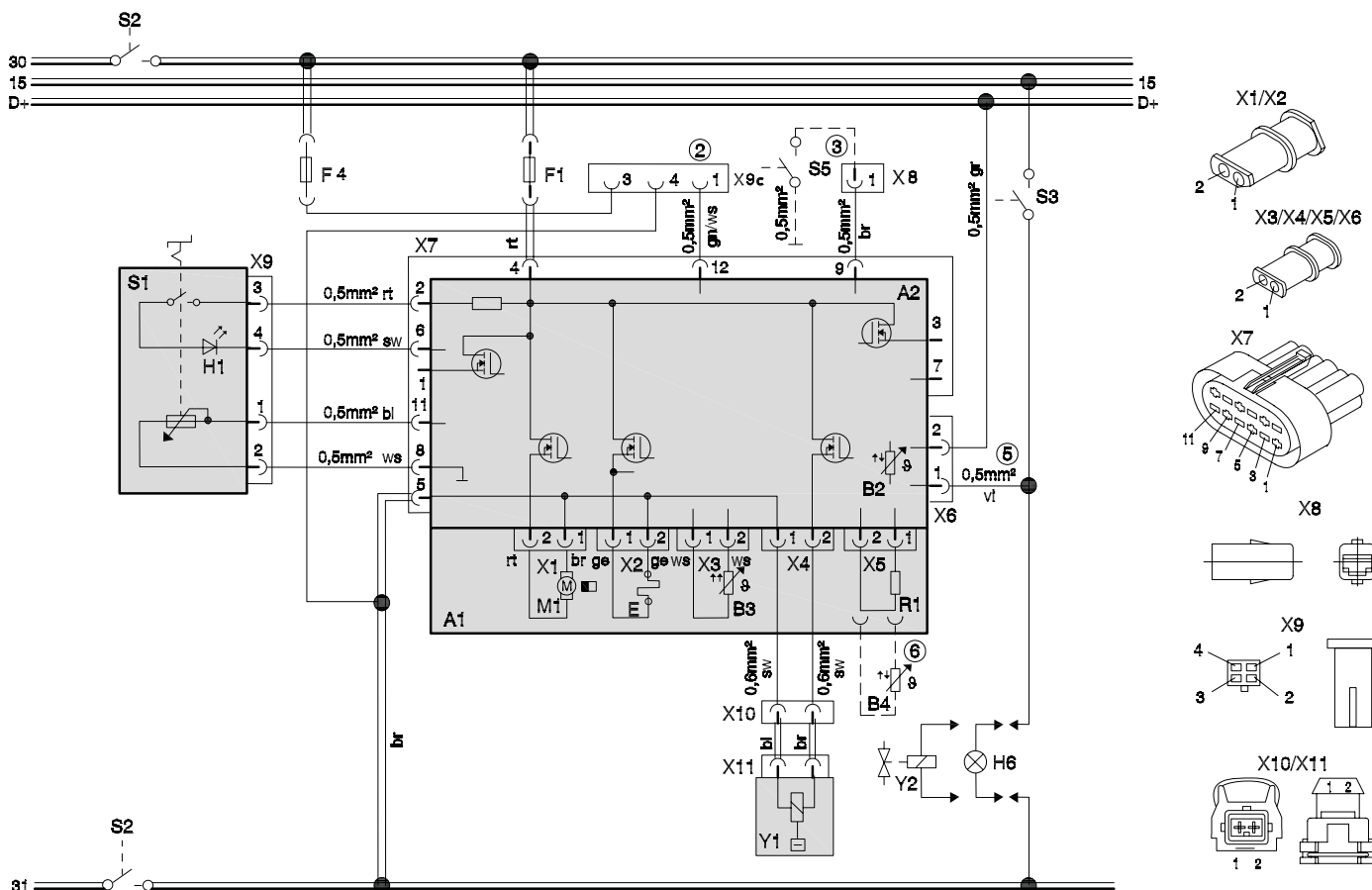
Fig. 703 Schéma électrique d'ensemble 24V, en mode ADR avec élément de commande
