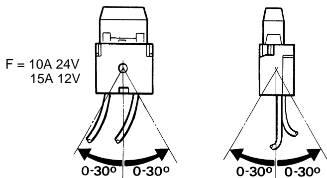
Fig. 811 Porte-fusibles, position de montage
