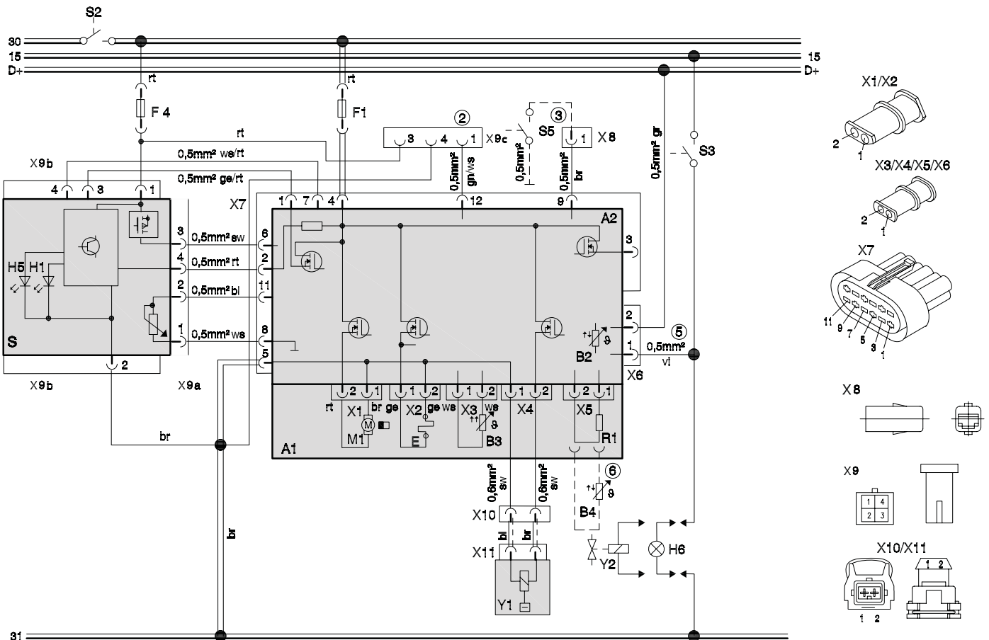
Fig. 707 Schéma électrique d'ensemble (diesel) 24V, en mode ADR avec élément de commande MC04/05
