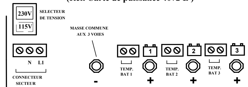
Figure B1 CONNECTIQUE TECPRO II, VERSION 97, 3 sorties (Réf. Carte de puissance 4072 E )
