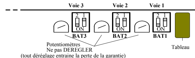
FIG. C - Position des interrupteurs pour la sélection du type de courbe de charge sur la carte de contrôle (Exemple de réglage courbe de charge profil B)
