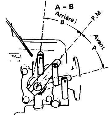
Commande d'inversion modèles KM2 et KM3
