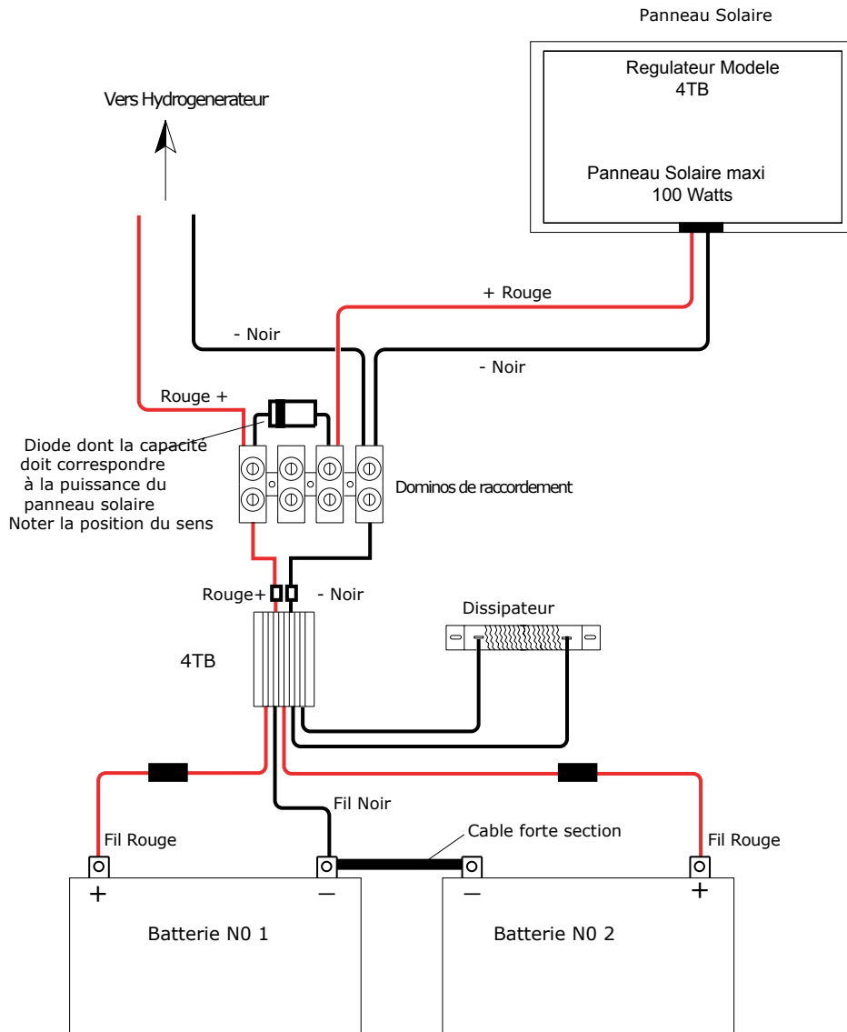
SCHEMA DE CABLAGE AVEC 4TB ET PANNEAU SOLAIRE REGULATION DE L'HYDROGENEUR AQ412 et D'un Panneau solaire de 100W
