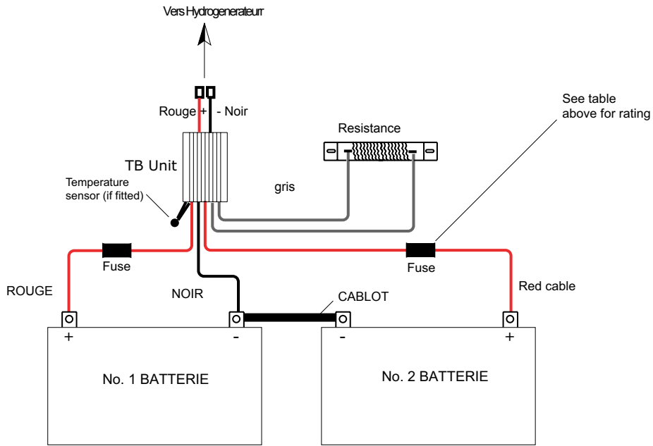
Schema de raaccordement pour deux parcs de batteries Séparées
