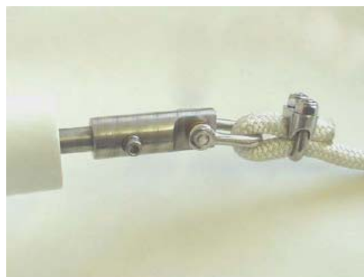
Raccordement du bout à l'accouplement Fig. 6
